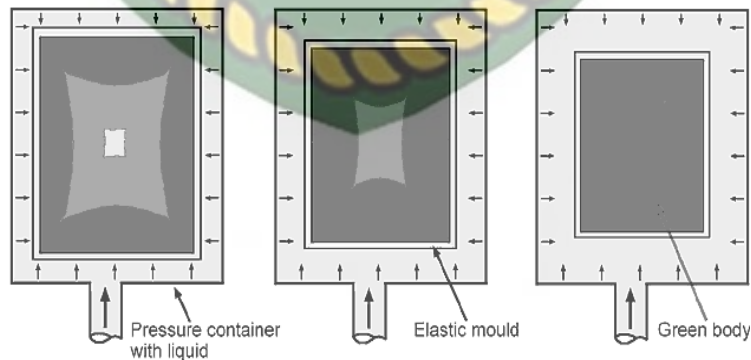
Gambar 2.8 Teknik Penekanan Iso-Statik
