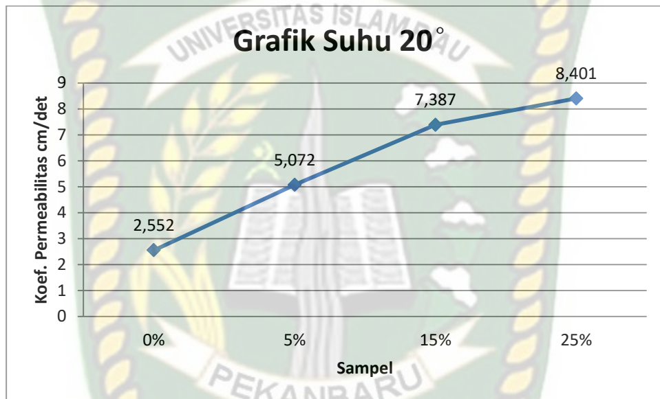
Gambar 5.7 Grafik Koefisien Permeabilitas Suhu Air 20°C
