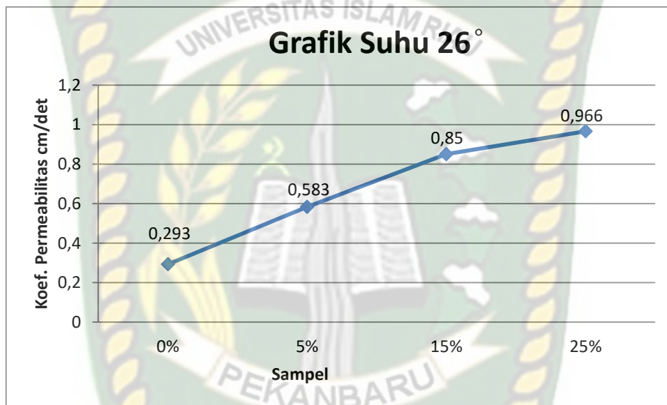
Gambar 5.6 Grafik Koefisien Permeabilitas Suhu Air 26^{\circ}\text{C}
