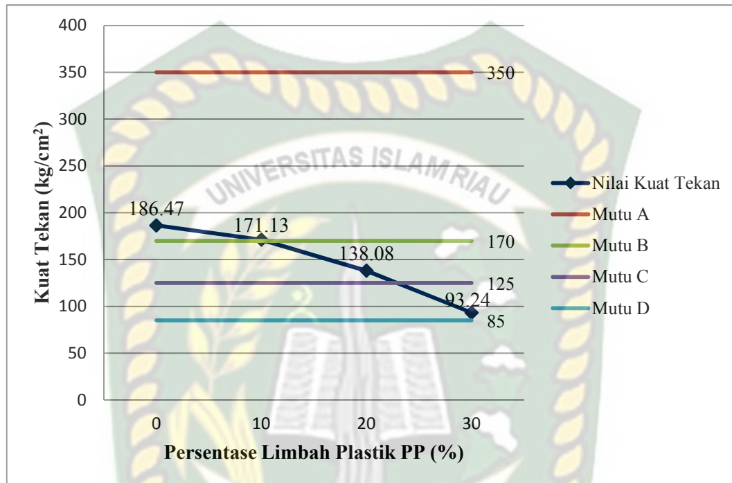
Gambar 5.3 Pengaruh Variasi Penggunaan Limbah Plastik PP Terhadap Kuat Tekan Paving Block
