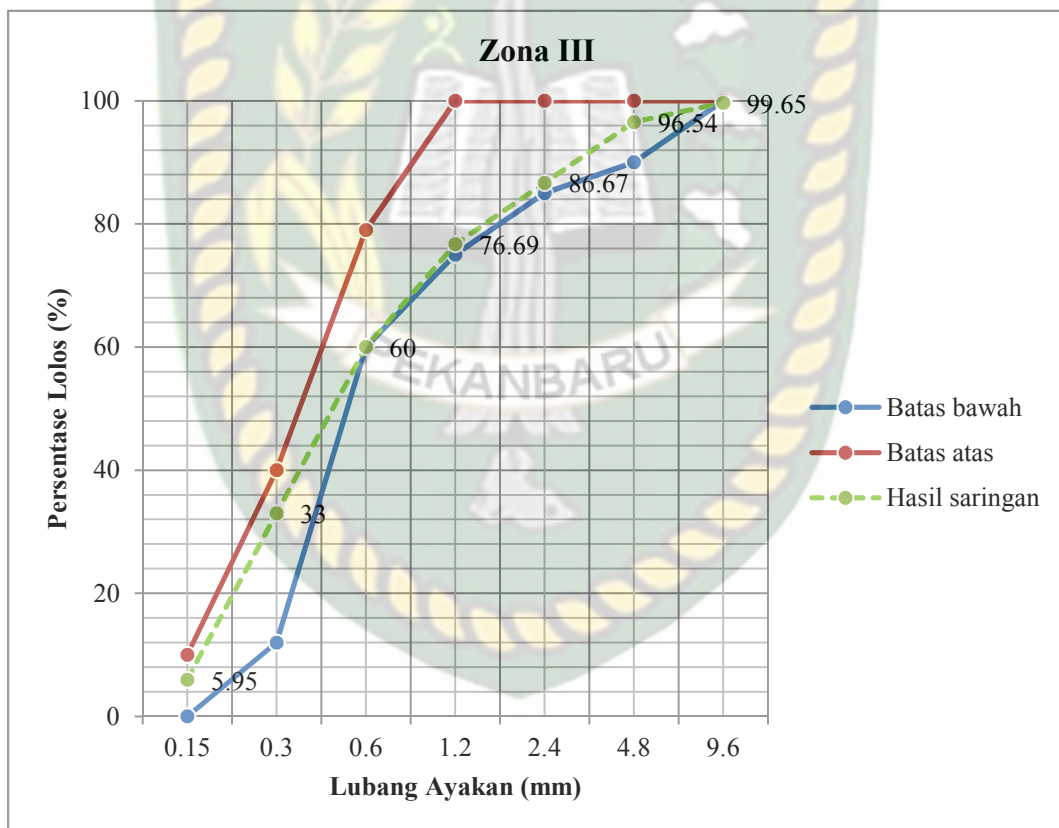
Gambar 5.1 Grafik Gradasi Pasir Pangkalan
