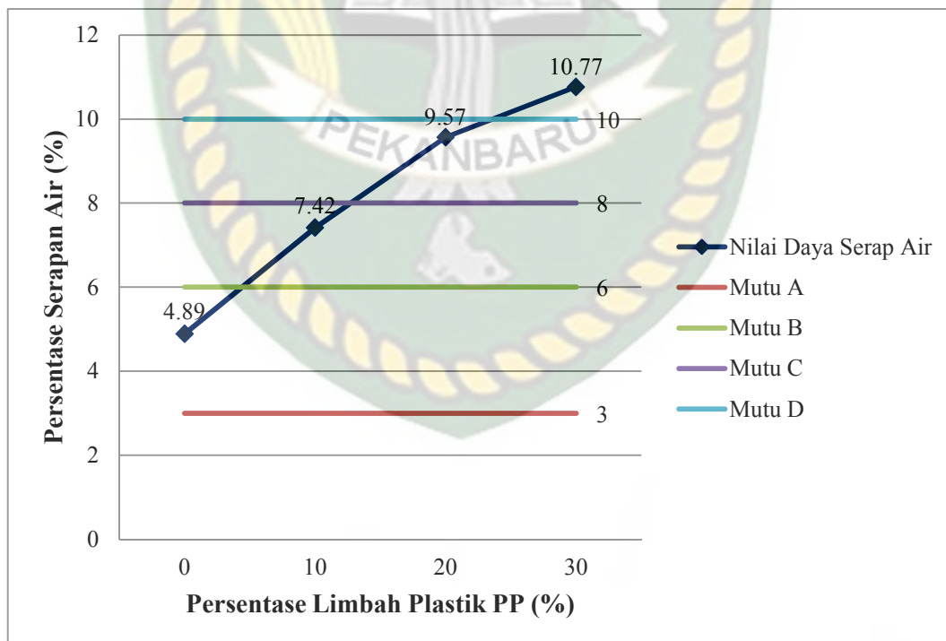
Gambar 5.5 Pengaruh Variasi Penggunaan Limbah Plastik PP Terhadap Daya Serap Air Paving Block
