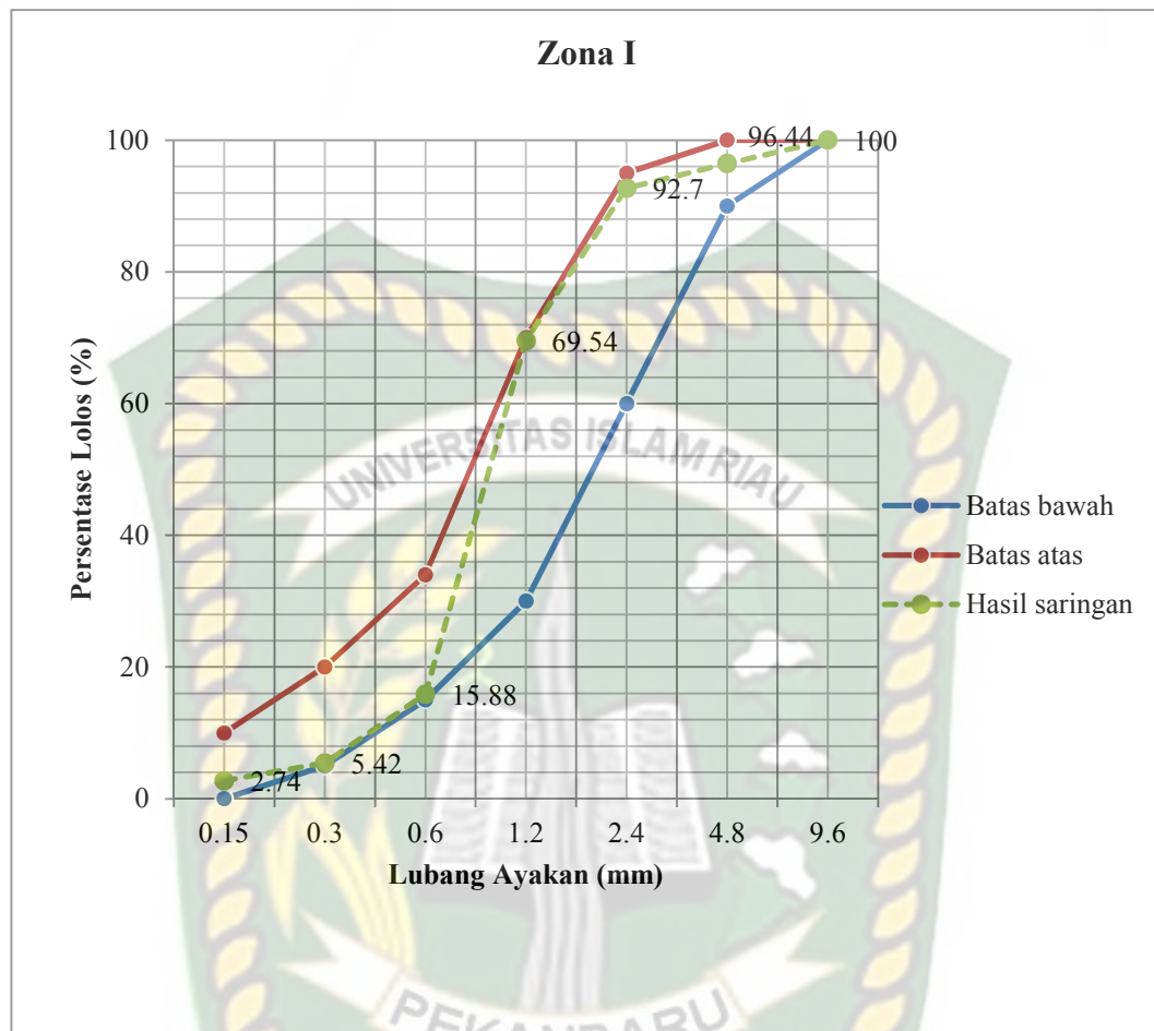
Gambar 5.2 Grafik Gradasi Limbah Plastik Polypropylene
