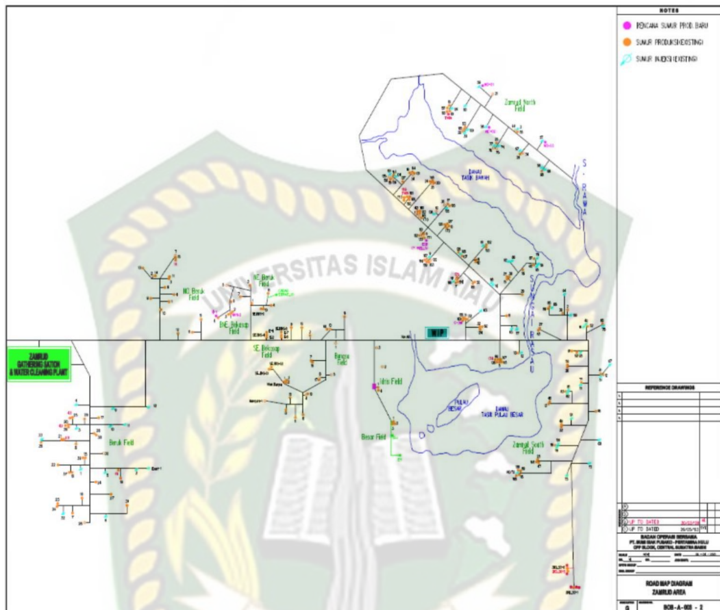
Gambar 3.2. Peta Sumur Produksi Lapangan Raya (BOB PT. BSP)
