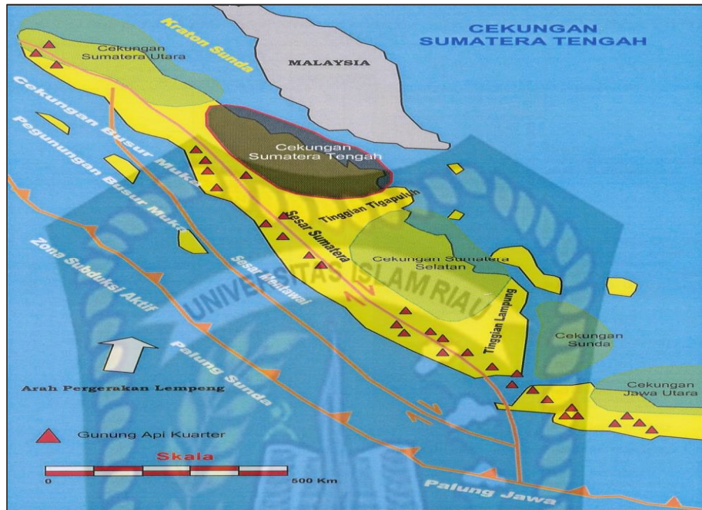
Gambar: 3.3 Tatanan Geologi Regional Cekungan Sumatera Tengah (Heidrick dan Aulia, 1993)
