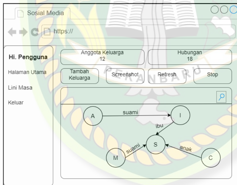
Gambar 3. 18 Desain Antarmuka Halaman Utama Pengguna
