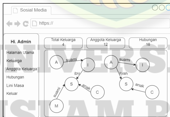
Gambar 3. 13 Desain Antarmuka Halaman Utama Admin
