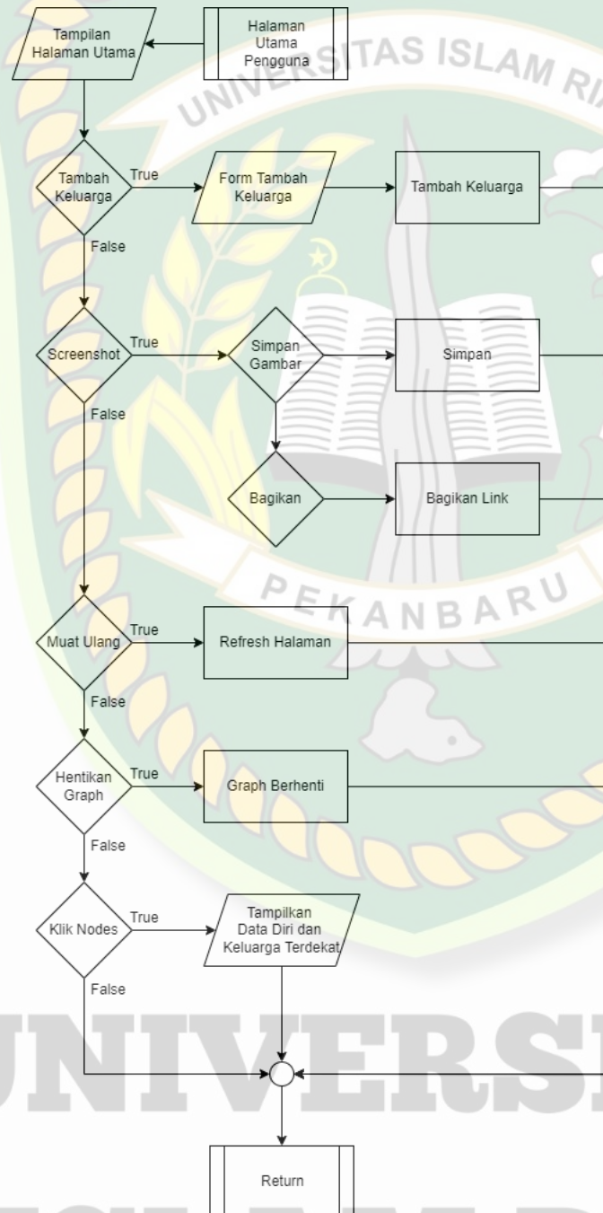
Gambar 3. 25 Flowchart Halaman Utama Pengguna
