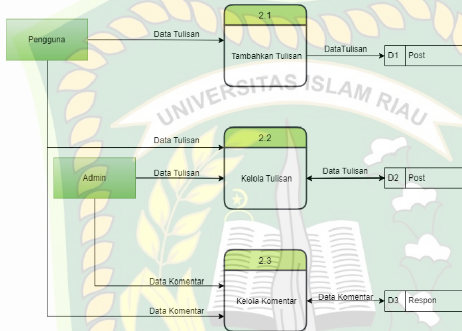
Gambar 3. 6 DFD Level 2
