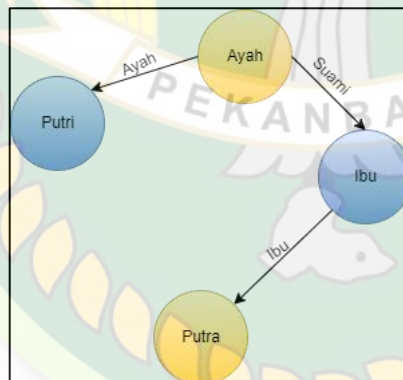
Gambar 2. 2 Graf Berarah
