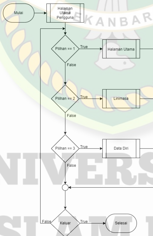
Gambar 3. 24 Flowchart Halaman Pengguna
