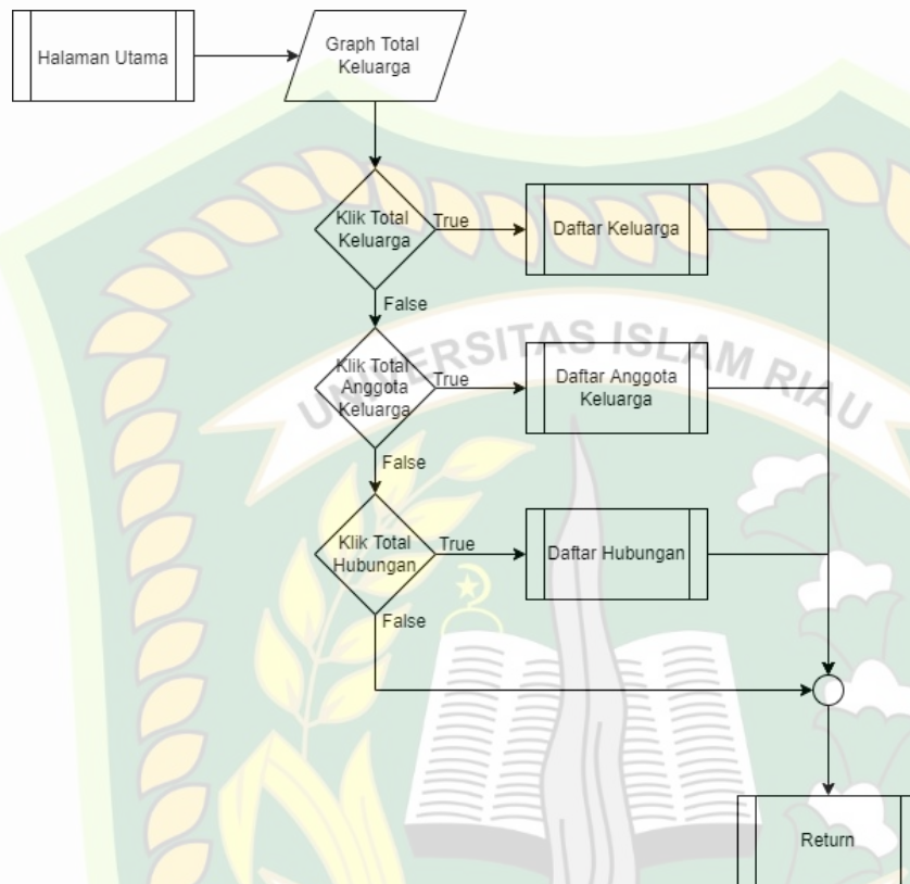
Gambar 3. 29 Flowchart Menu Halaman Utama
