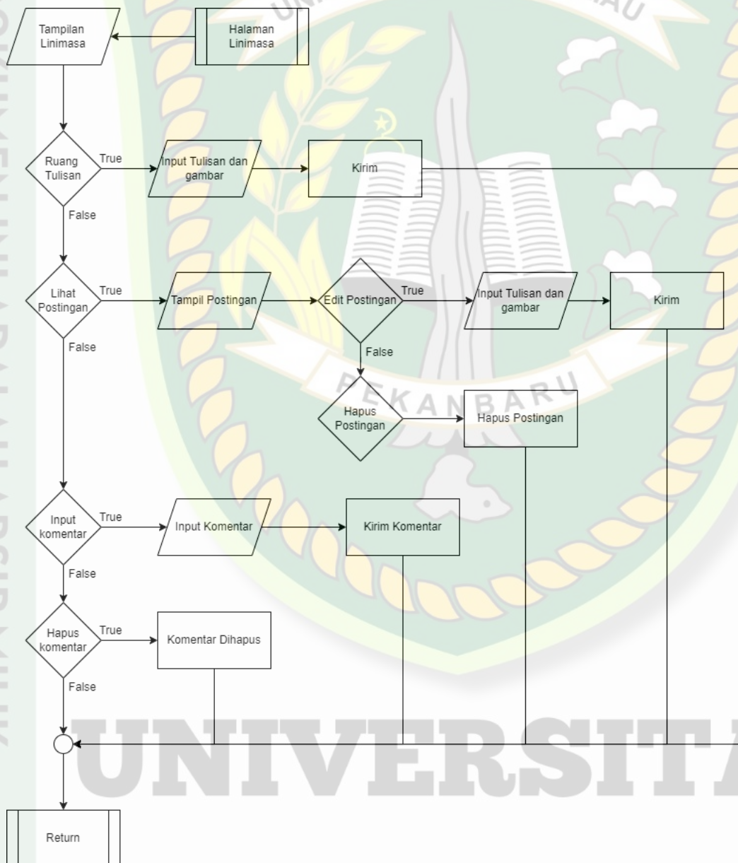
Gambar 3. 26 Flowchart Halaman Linimasa Pengguna
