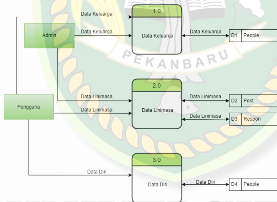
Gambar 3. 5 DFD Level 1
