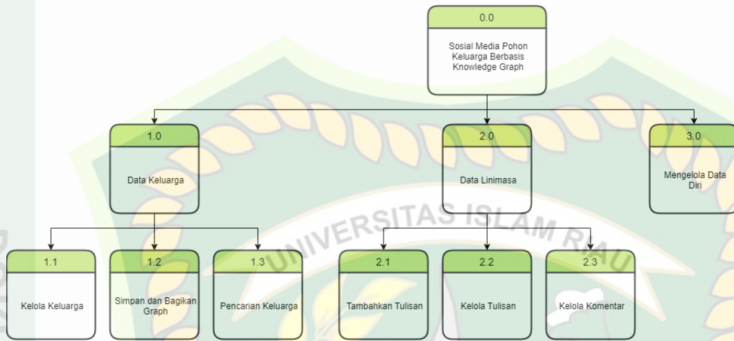
Gambar 3. 3 Hierarchy Chart Sosial Media Pohon Keluarga
