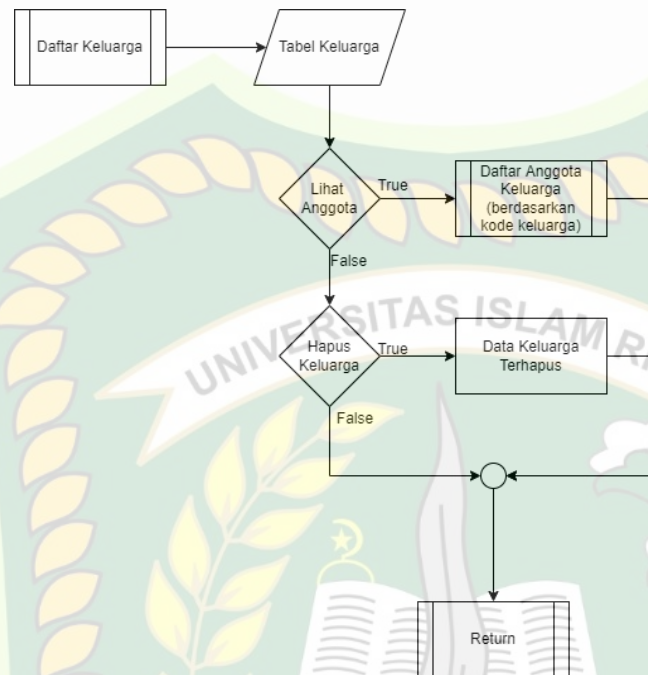
Gambar 3. 30 Flowchart Menu Halaman Daftar Keluarga
