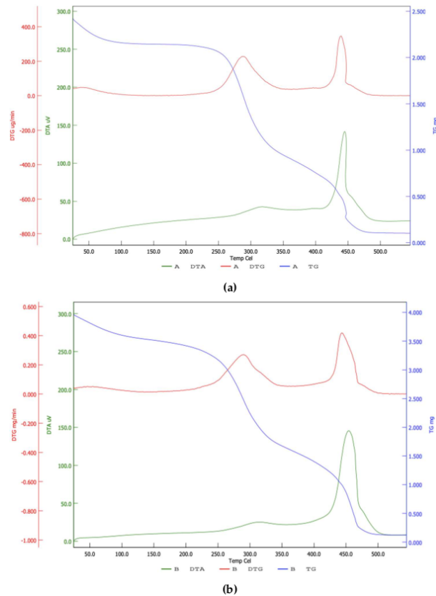
Gambar 3 Hasil TG/DTG Briket Sabut Kelapa pada suhu 30°C-550°C (a) Sabut Kelapa Tua; (b) Sabut Kelapa Muda
