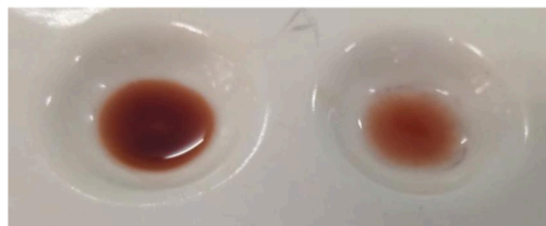
Gambar 3. Uji steroid dan terpenoid
