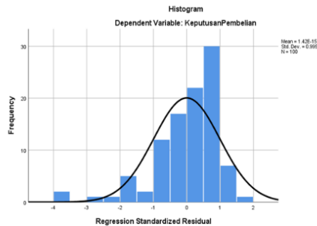
Gambar 1. Uji Histogram
