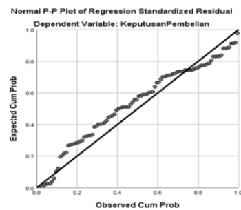
Gambar 2. Pengujian Normal P-Plot
