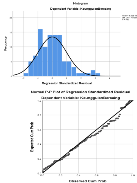
Gambar 1. Normalitas Data
