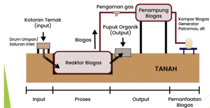
Gambar 1. Cara sederhana pembuatan Biogas Rumah Tangga
