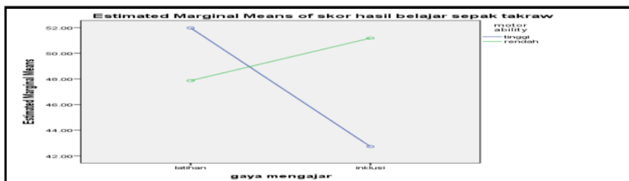
Gambar 1. Interaksi A*B
