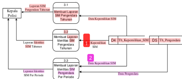
1 Gambar 4. DFD Level 1 Proses 3 Legalitas Surat Izin Mengemudi (SIM)
