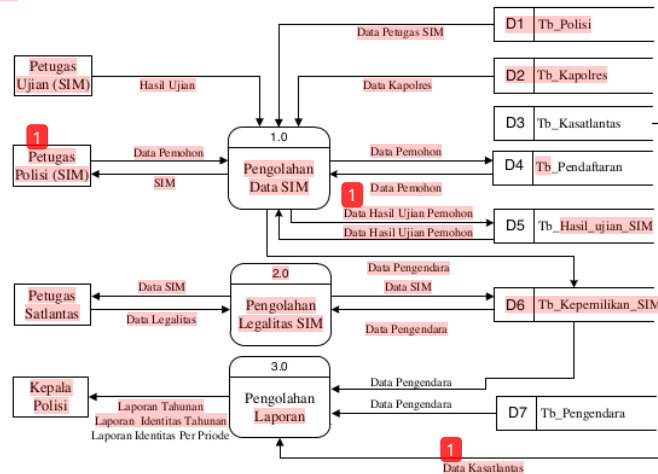
Gambar 2. DFD Level 0 Legalitas Surat Izin Mengemudi (SIM)
