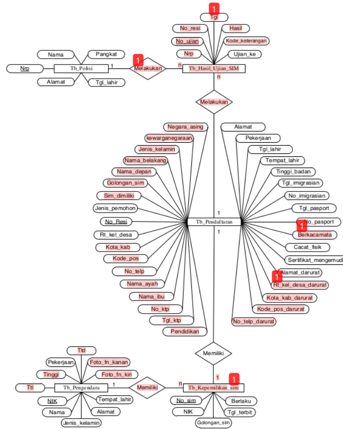
Gambar 5. ERD Legalitas surat Izin Mengemudi (SIM)
