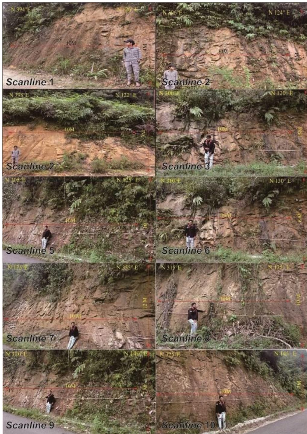
Gambar 4: Scanline pengukuran diskontinuitas di lokasi penelitian
