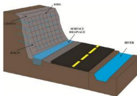
Gambar 5: Hasil pemodelan lereng daerah penelitian
