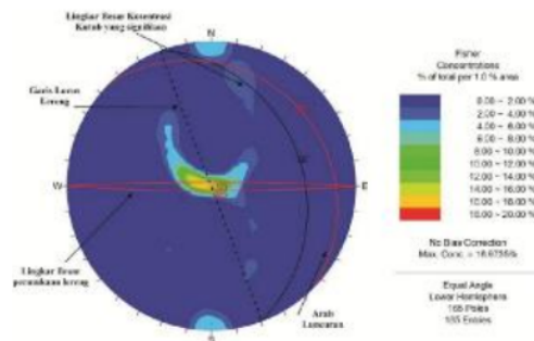
Gambar 5: Hasil plot data-set diskontinuitas
