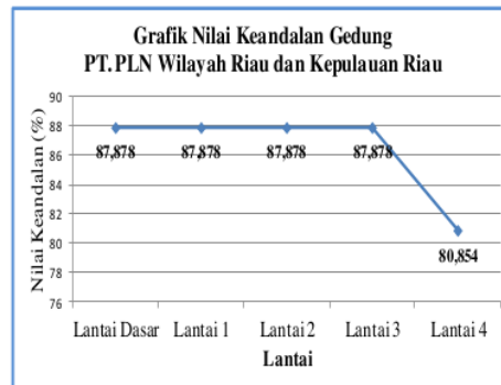
Gambar 4 Grafik Nilai Keandalan Gedung PT. PLN Wilayah Riau dan Kepulauan Riau
