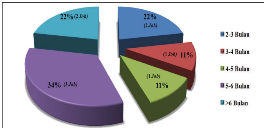
Figure 5 Long Cyclic Heat Endurance Time (HET) (Januari 2013 - Oktober 2016).
