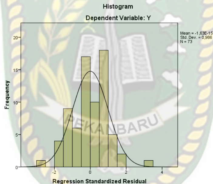
Gambar 5.1 Grafik Histogram
