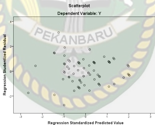
Gambar 5.3 Grafik Scatterplot
