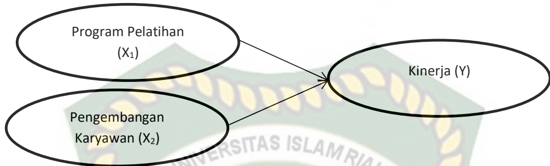
Gambar 2.1 Kerangka Penelitian
