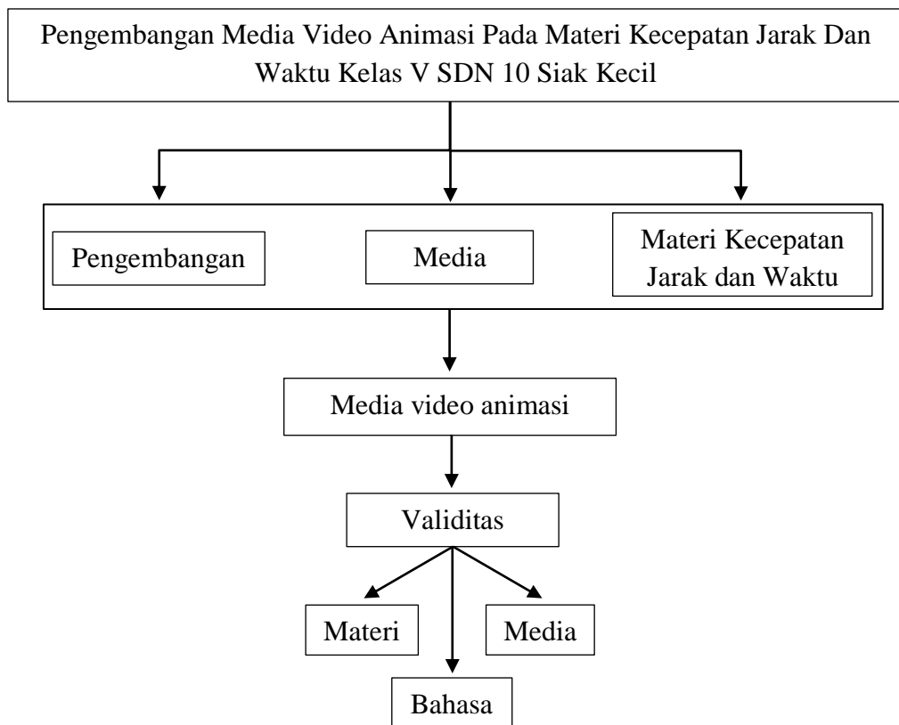
Gambar 2.1 Kerangka Berpikir
