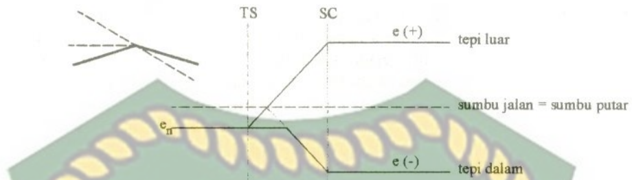
Gambar 3.3. Diagram super elevasi dengan sumbu jalan sebagai sumbu putar
