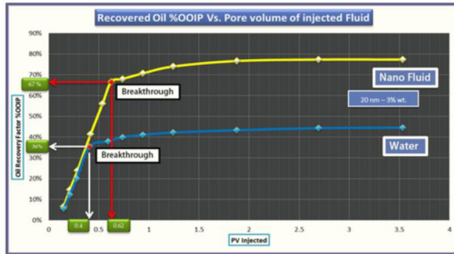
Gambar 3. Volume pori injeksi versus Perolehan minyak [7].
