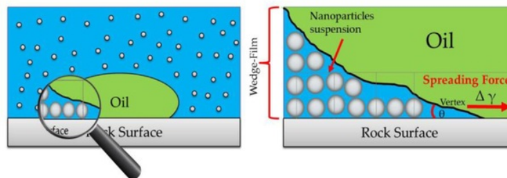
Gambar 2. Mekanisme nanoparticles dalam skala micro [7].
