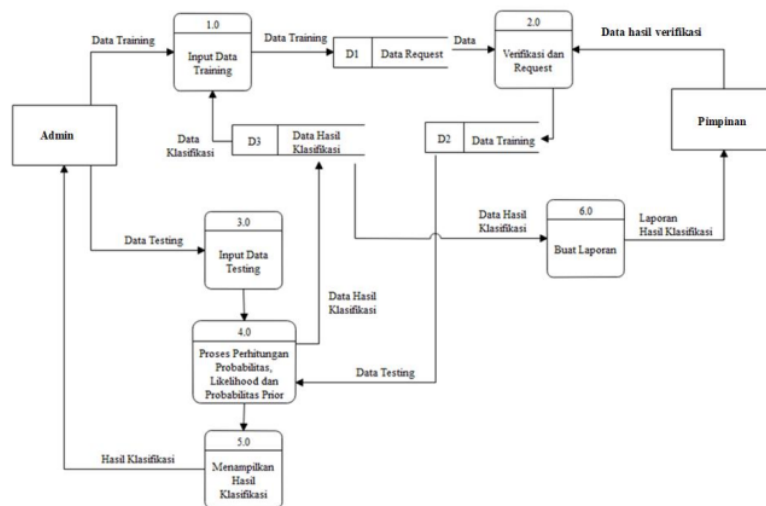
Gambar 3. DFD Sistem Klasifikasi Kualitas Produk Kelapa Sawit
